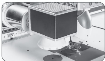
V— 激光振镜热雕装置 V—laser galvanometer hot engrave
